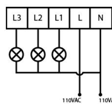
CONEXIÓN A 220 VOLTIOS
