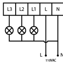
CONEXIÓN A 110 VOLTIOS
